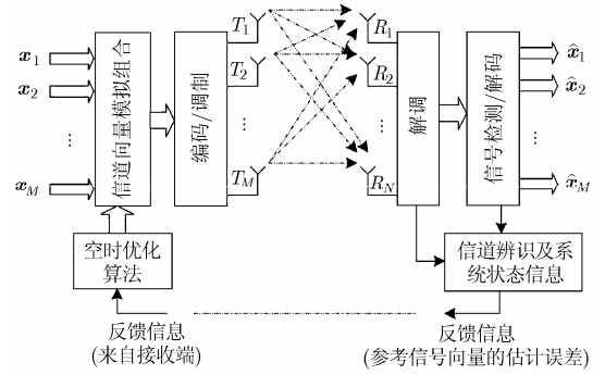
图1 协同信道空时优化 MIMO 无线传输系统的基本结构
