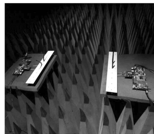
图 5 实验测试环境(微波暗室)
