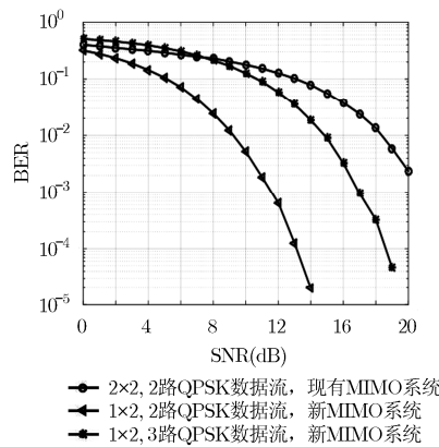
图 3 1 发 2 收 2 路 QPSK 数据流和 3 路 QPSK 数据流的新 MIMO 系统和 2 发 2 收 2 路 QPSK 数据流的现有 MIMO 系统的 BER 性能比较
