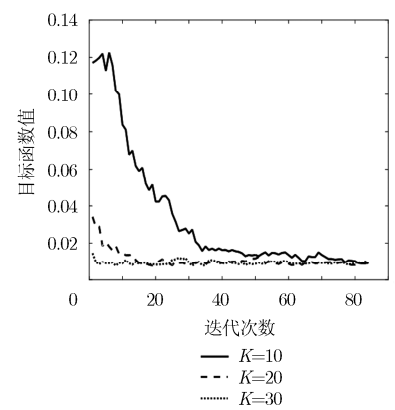
图 4 2 发 2 收 2 路 QPSK 数据流的新 MIMO 系统中,采用不同内循环次数的模拟退火算法的收敛特性
