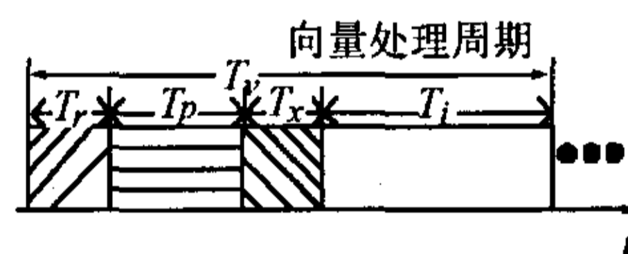
图 3 SAR 信号处理的向量处理时序
