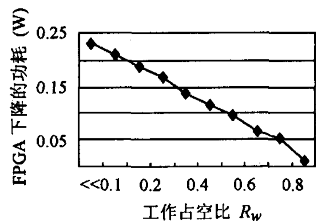
图9 使用 Clock-gating 后 FPGA 下降的功耗与工作占空比的关系
