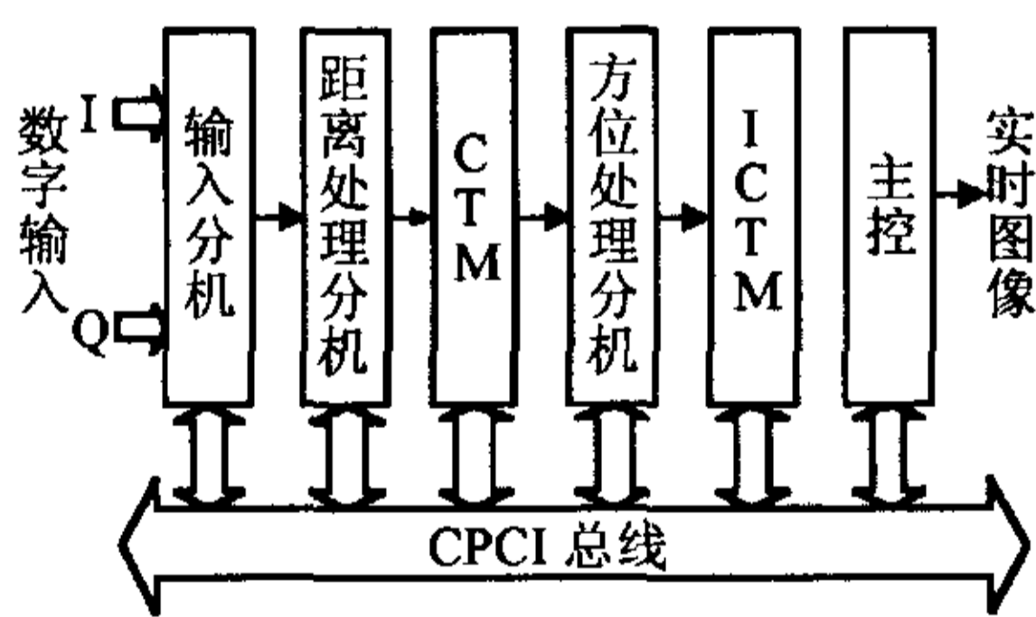
图 2 典型 SAR 实时成像系统的体系结构
