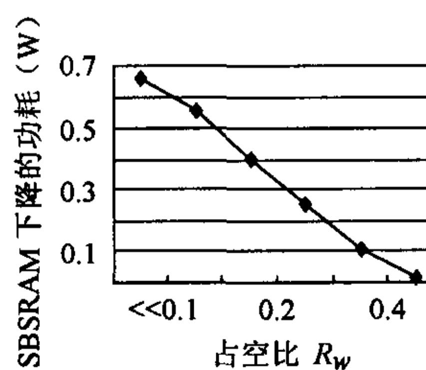
图8 采用 Clock-gating 后 SBSRAM 下降的功耗与工作占空比的关系
