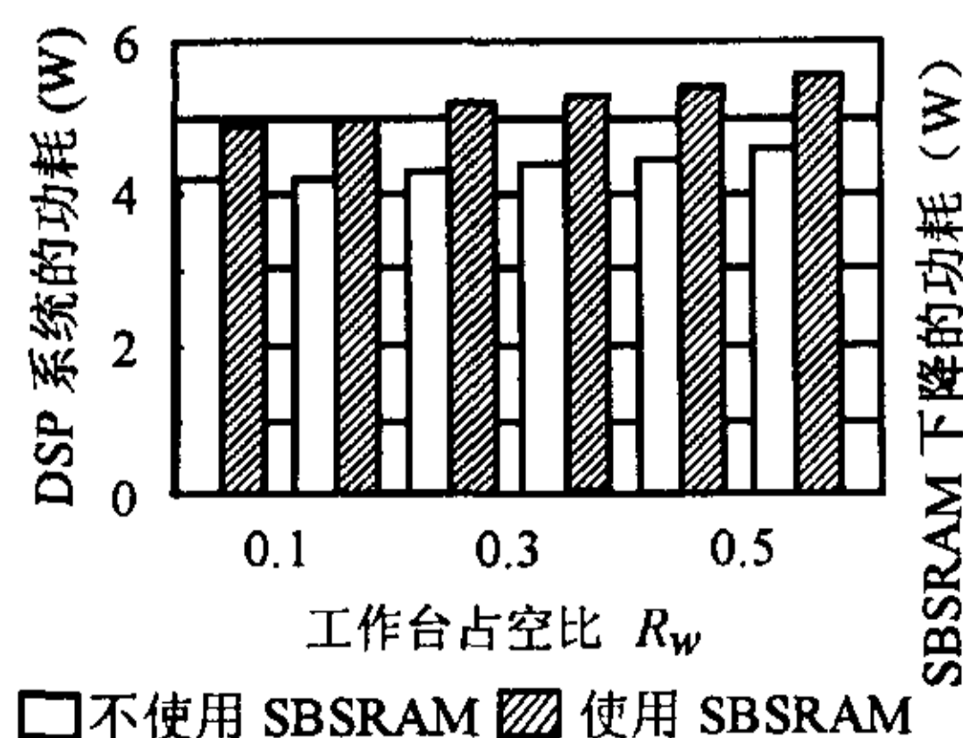
图7 使用 SBSRAM 前后, DSP 系统功耗与占空比的关系
