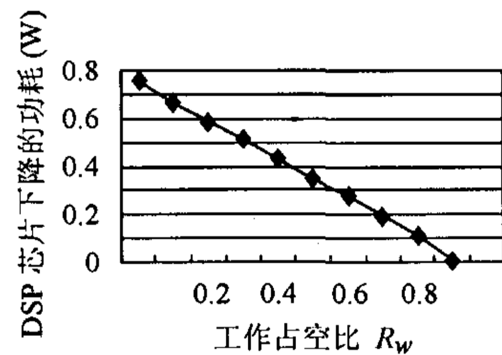
图6 采用 Clock-gating 后 DSP 芯片下降的功耗与工作占空比的关系
