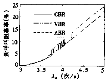
图 6 应用动态容量分配算法时小区 1.1 空中接口各类新呼叫阻塞率随新呼叫瞬时发生率变化曲线
