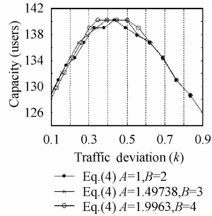
图5 嵌入波束结构系统容量随k变化图 Fig.5 Capacity vs. k of embedded beams
