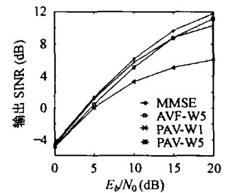
图 2 有同步失调时接收机性能随着 E_b/N_0 变化
