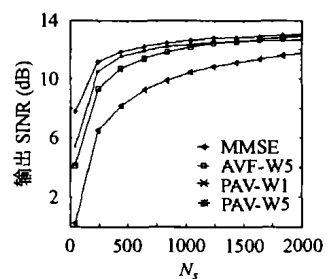
图 4 接收机性能随着符号数变化
