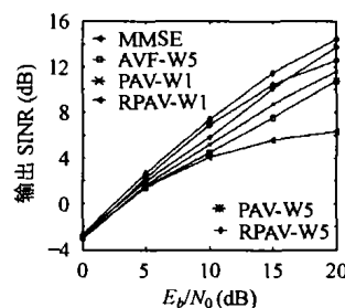
图 3 接收机性能随着 E_b/N_0 变化
