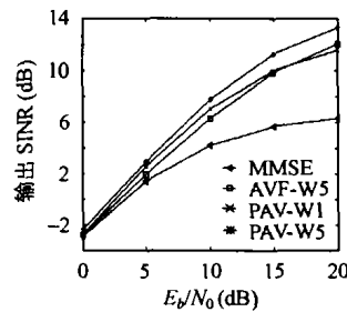
图 1 没有同步失调时接收机性能随着 E_b/N_0 变化
