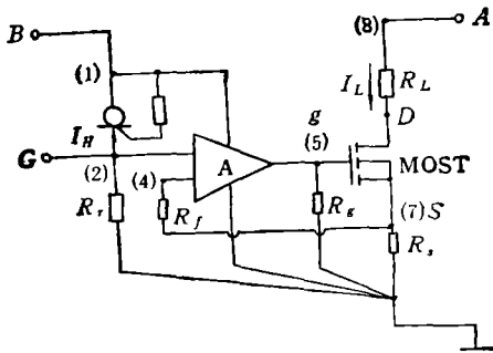
图 2 基本电路图
