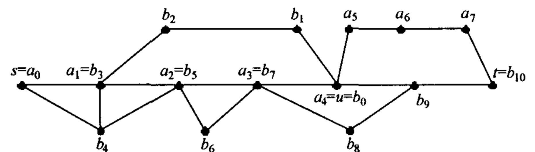
图 1 r = p ⊕ q 示例
