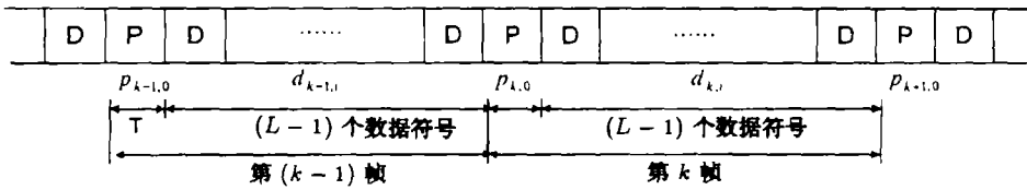
图 2 信号的帧结构
