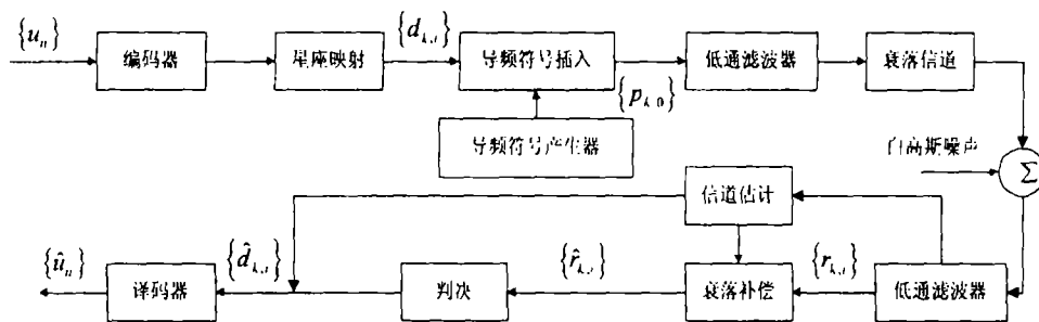
图 1 系统框图
