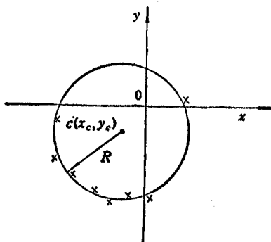
图1 复平面上的输入反射系数圆
