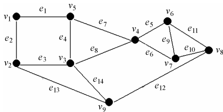
图2 网络图 G Fig.2 Network graph G
