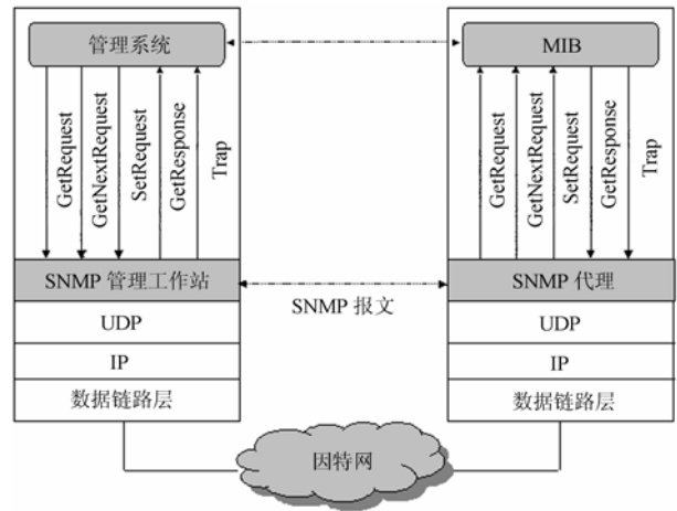
图 1 SNMP 原理
