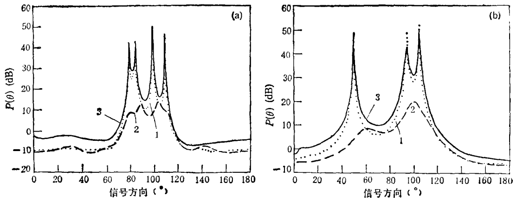
(a) 四个信号 (SNR 均为 25dB) 来自 80^\circ, 85^\circ, 100^\circ 和 110^\circ 方向
