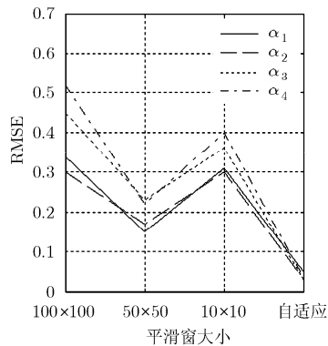
(b) 参数 \alpha_i 估计误差
