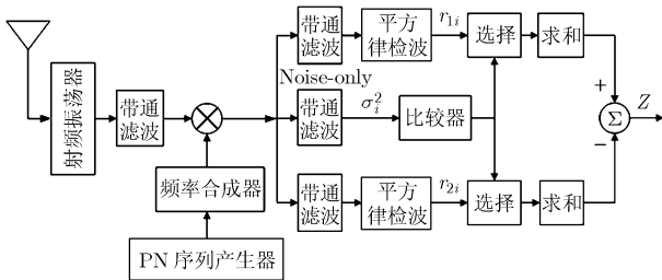
图 1 FH/BFSK 系统选择分集合并接收机模型
