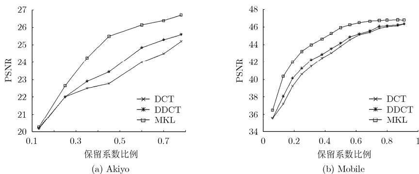
图 5 视频预测残差 M-KL 变换编码与 DCT 和 DDCT 编码的结果比较
