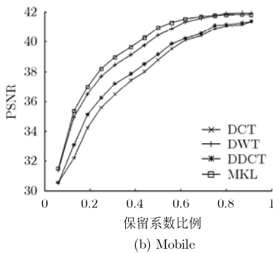
图 2 静态图像 M-KL 变换编码与 DCT, D-DCT 和 DWT 编码的结果比较
