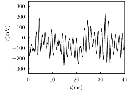
图 7 雷达工作在 CW 模式时的中频信号时域波形
