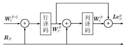
图 3 乘积码软译码简化框图
