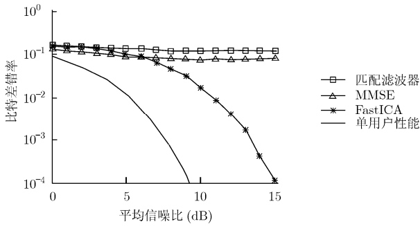
图 2 20 用户的平均比特差错率曲线
