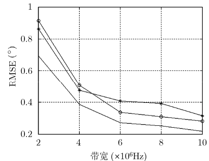
图 2 角度估计性能随信号带宽变化情况
