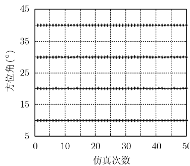
图 3 信源过载时算法的方位估计曲线
