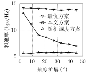
图3 各方案的平均吞吐量 ( \rho=0.2, K=20, SNR=10dB )
