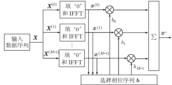
图 1 PTS 算法的实现框图
