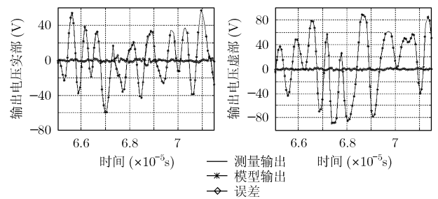
图2 Volterra-Laguerre 模型 K=2 , L=3 时测量和模型输出电压的波形比较
