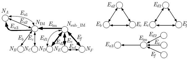
图 9 子会议 REL
