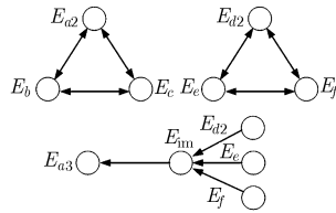
图 10 子会议 RL
