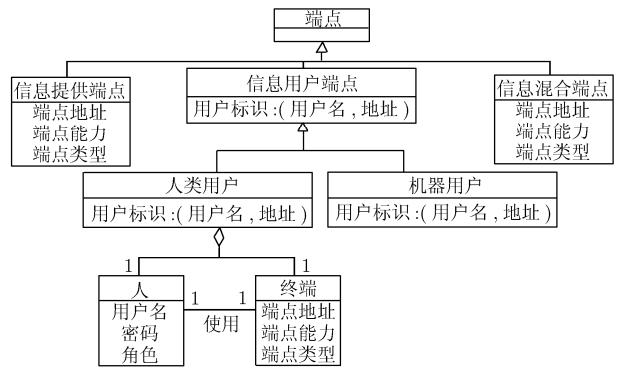
图 2 端点对象图
