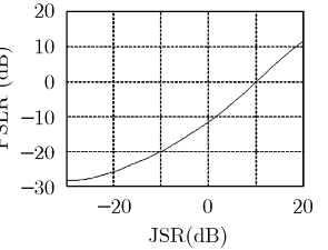
图4 干扰作用下相关输出的 PSLR 随 JSR 的变化趋势
