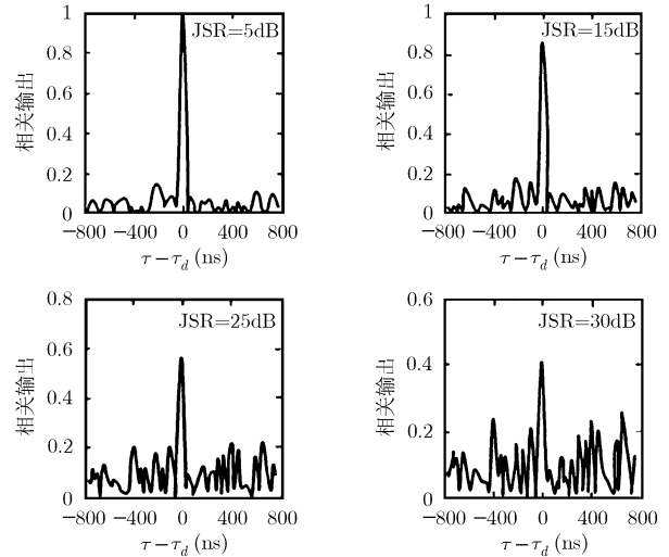
图11 抗干扰后归一化相关输出
