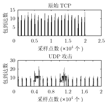
图1 正常 TCP 和包含 UDP 攻击的统计流量对比
