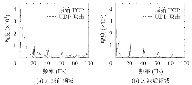
图4 过滤前后的频谱对比
