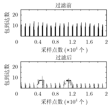
图5 时域中含 UDP 攻击流量过滤前后的比较
