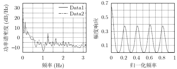
图2 正常 TCP 和包含 UDP 攻击的流量 PSD 对比
