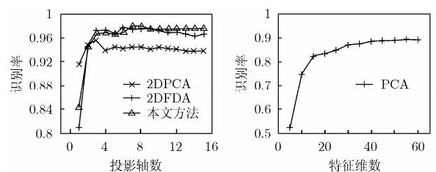
图 3 不同方法在维数变化情况下的识别率
