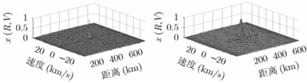
图 9 \theta_R=85^\circ 时的模糊图 图 10 \theta_R=-85^\circ 时的模糊图
