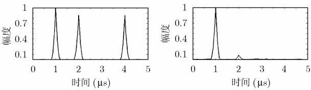
图 11 匹配滤波输出(无频移) 图 12 匹配滤波输出(有频移)
