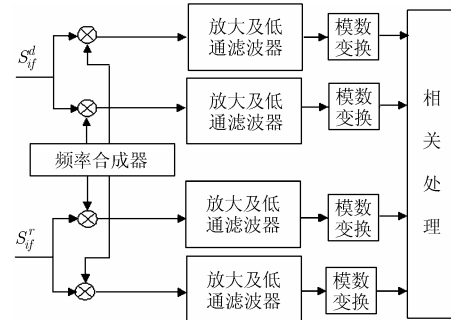
图 2 基频信号的相关处理
