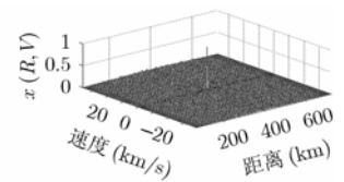
图 6 \theta_R = -10^\circ 时的模糊图
