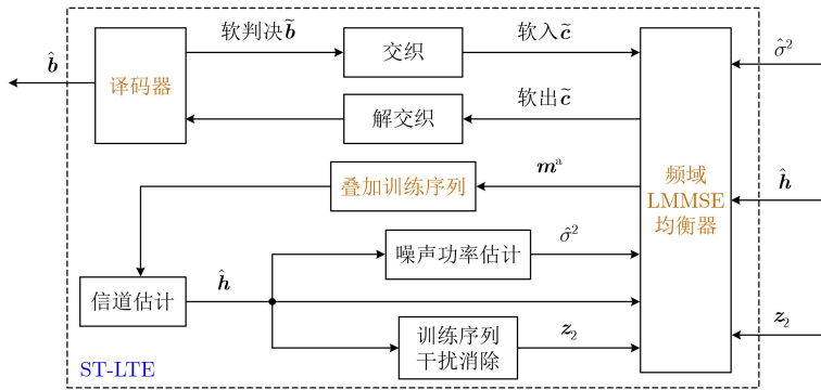
图2 Turbo均衡
