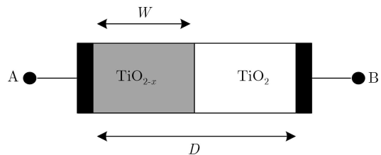
图1 HP忆阻器的结构图
