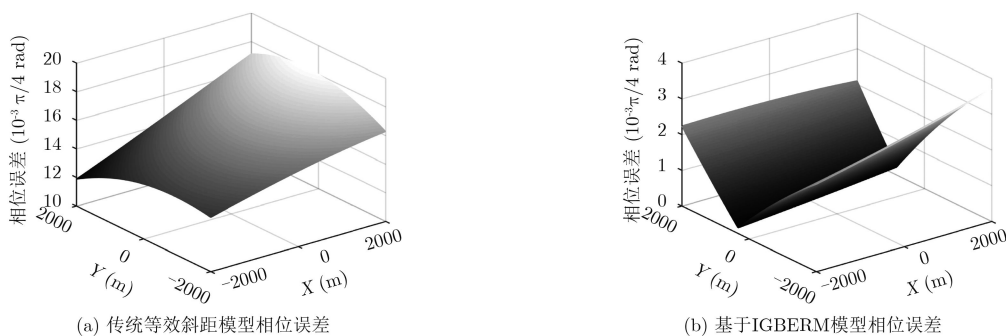
图3 相位误差结果对比
