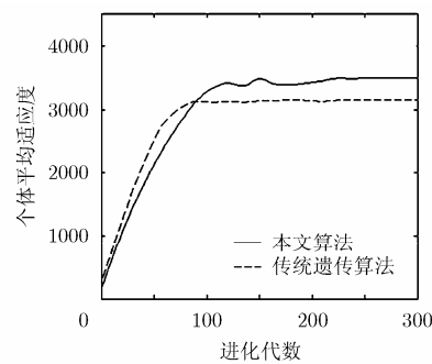
图 7 传统与改进遗传算法的 ONU-BS 规划算法比较
