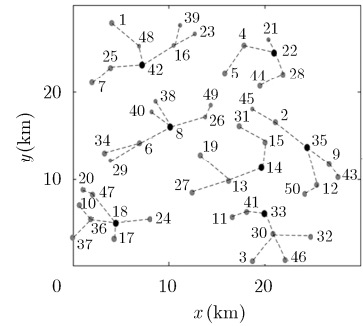
图 5 基站数量 50 的规划结果
