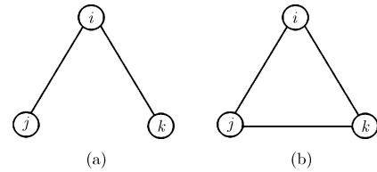
图1 以点 i 为一个顶点的三元组的可能两组形式
