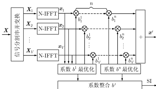
图2 多级寻优的PTS原理框图
