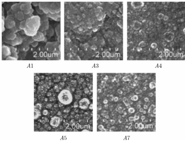
图 6 各种 PPy 膜的 SEM 照片(放大两万倍)
