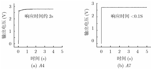
图 5 芯片响应时间
