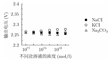
图 7 芯片对不同盐溶液的响应
