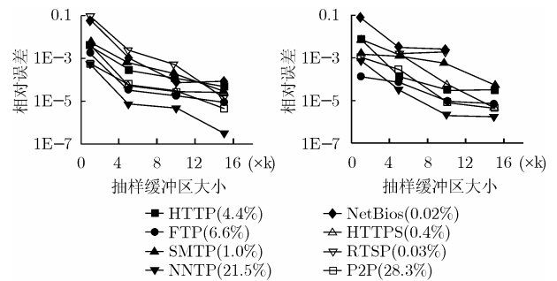
图 5 缓冲与相对误差关系(aflow1)
