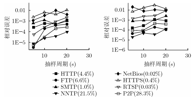
图 7 T 对相对误差的影响(aflow1)
