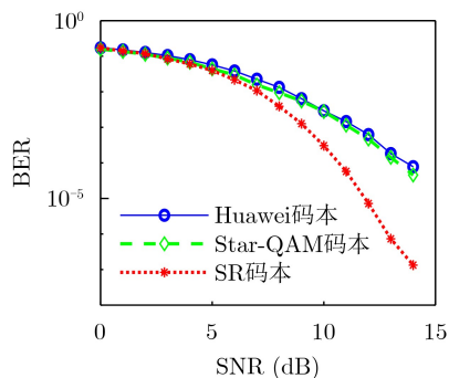
图4 传统SCMA系统各码本性能对比图
