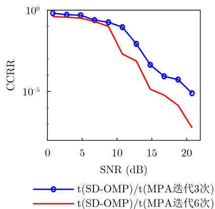
图5 多用户检测算法仿真CCRR对比图
