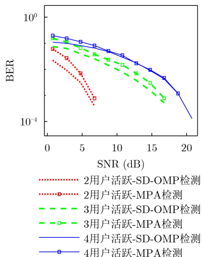
图6 部分用户活跃时检测算法性能仿真曲线
