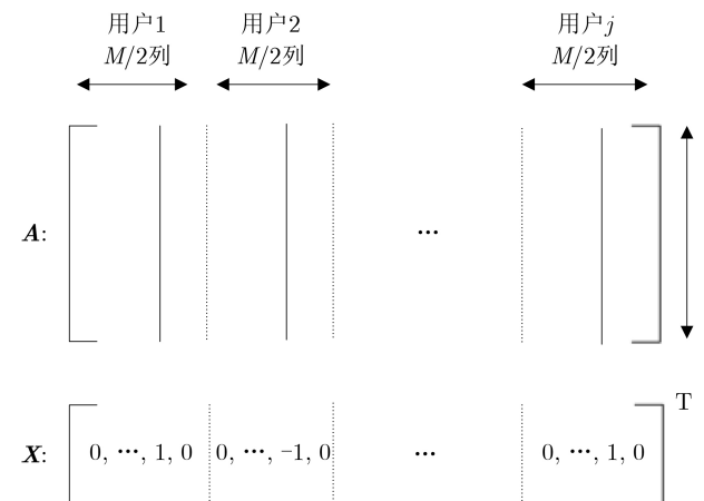
图3 稀疏信号重构模型
