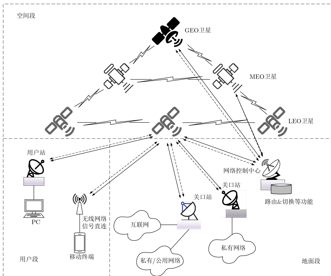
图1 卫星通信系统架构
